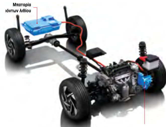
Ηλεκτροκινητήρας MGU
